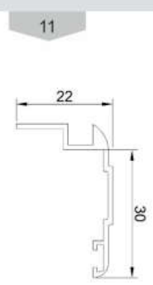
روکوب ۳۰ Suppressed the binding Code : 10023 weight : 0.23 kg/m
