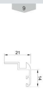
روکوب ۱۴ Suppressed the binding Code : 10021 weight : 0.2 kg/m
