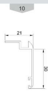
روکوب ۳۰ Suppressed the binding Code : 10022 weight : 0.22 kg/m
