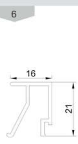
زهوار دو جداره Double rickety Code : 12352 weight : 0.23 kg/m
