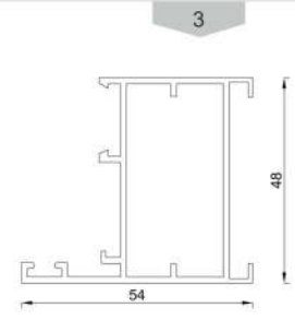
پروفیل فریم Frame profile Code : 12312 weight : 0.8 kg/m
