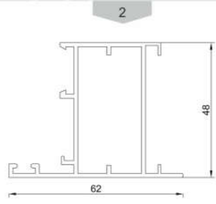
پروفیل فریم Frame profile Code : 12311 weight : 0.84 kg/m
