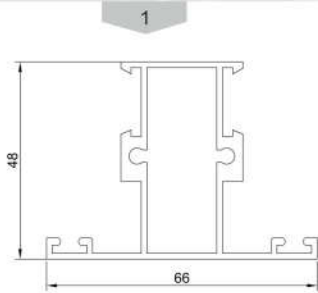
پروفیل سپری T profile Code : 12341 weight : 1 kg/m
