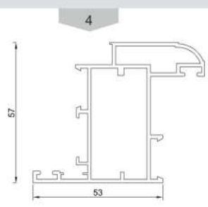
پروفیل لنگه Vent profile Code : 12331 weight : 1.1 kg/m
