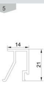
زهوار دوجداره Double rickety Code : 12351 weight : 0.22 kg/m
